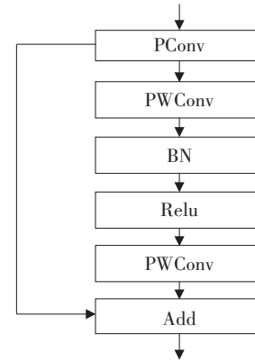
图 2 FasterNet 块
