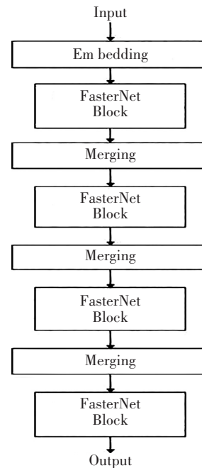
图 3 改进的主干网络
