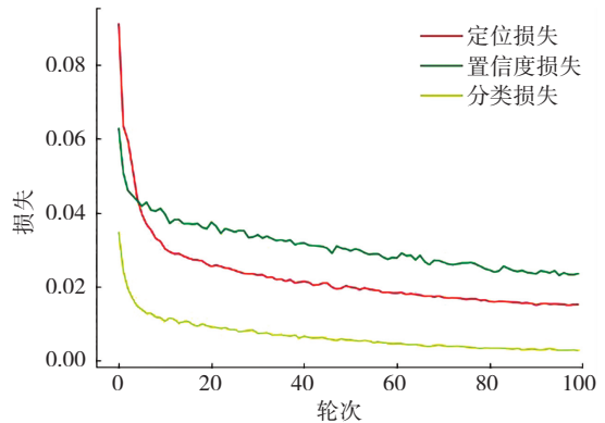
图 5 损失函数变化图
