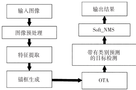
图 4 改进后的苹果检测算法流程图
