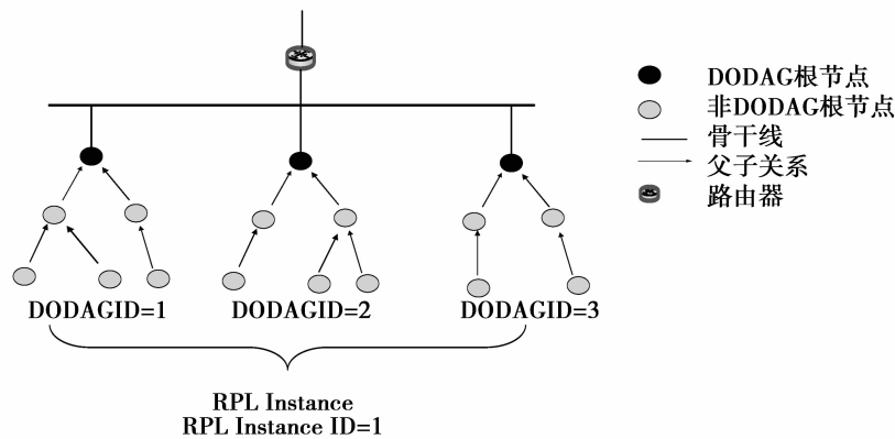
图 2 RPL Instance
