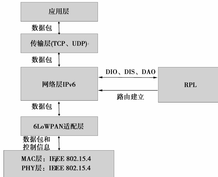
图 1 6LoWPAN 协议体系
