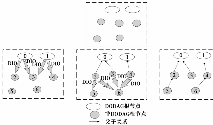
图 5 路由协议建立过程描述
