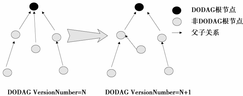
图 3 DODAGVersionNumber
