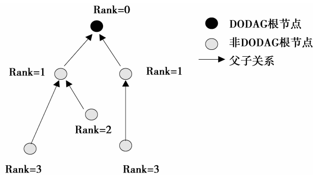
图 4 DODAG Rank 值
