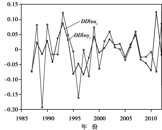
图 4 \nabla^2 \ln x_t 和 \nabla^2 \ln y_t 图
