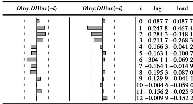
图 5 \{\nabla \ln y_t\} 和 \{\nabla^2 \ln x_t\} 的相互关系图
