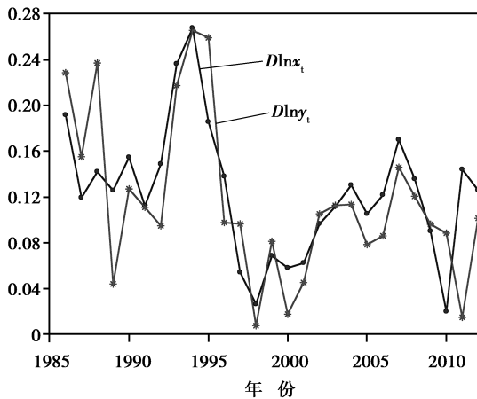
图 3 \nabla \ln x_t 和 \nabla \ln y_t
